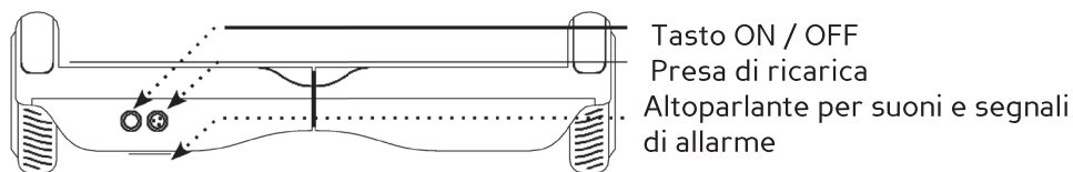
Figura. 4.2.D. • caricabatteria
